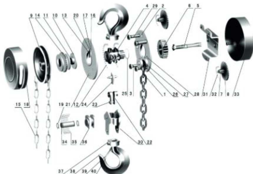
Рис. 5 Схема сборки
